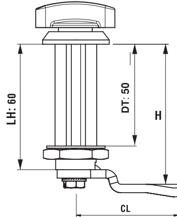
064 362-DT-1-2-CC ЗАМАК – ЧЕРНОЕ ПОКРЫТИЕ
