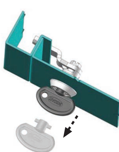
Ключ извлекается в закрытом положении
