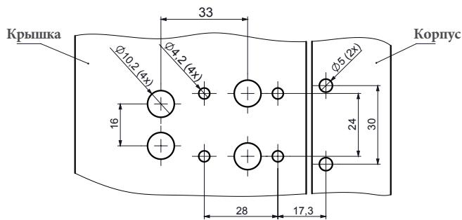
Монтажные отверстия
