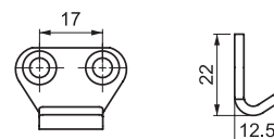
Фиксирующая планка
