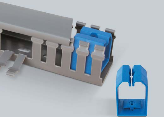
Kablo Tutucu Aparatı Cable Holder Apparatus
